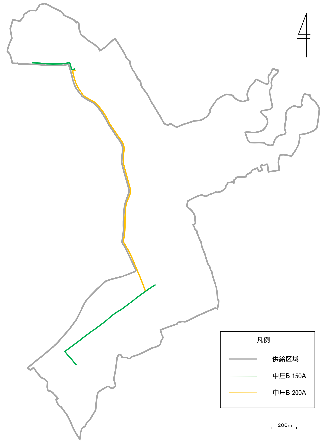
第8表 主要導管圖(里庄地区)
